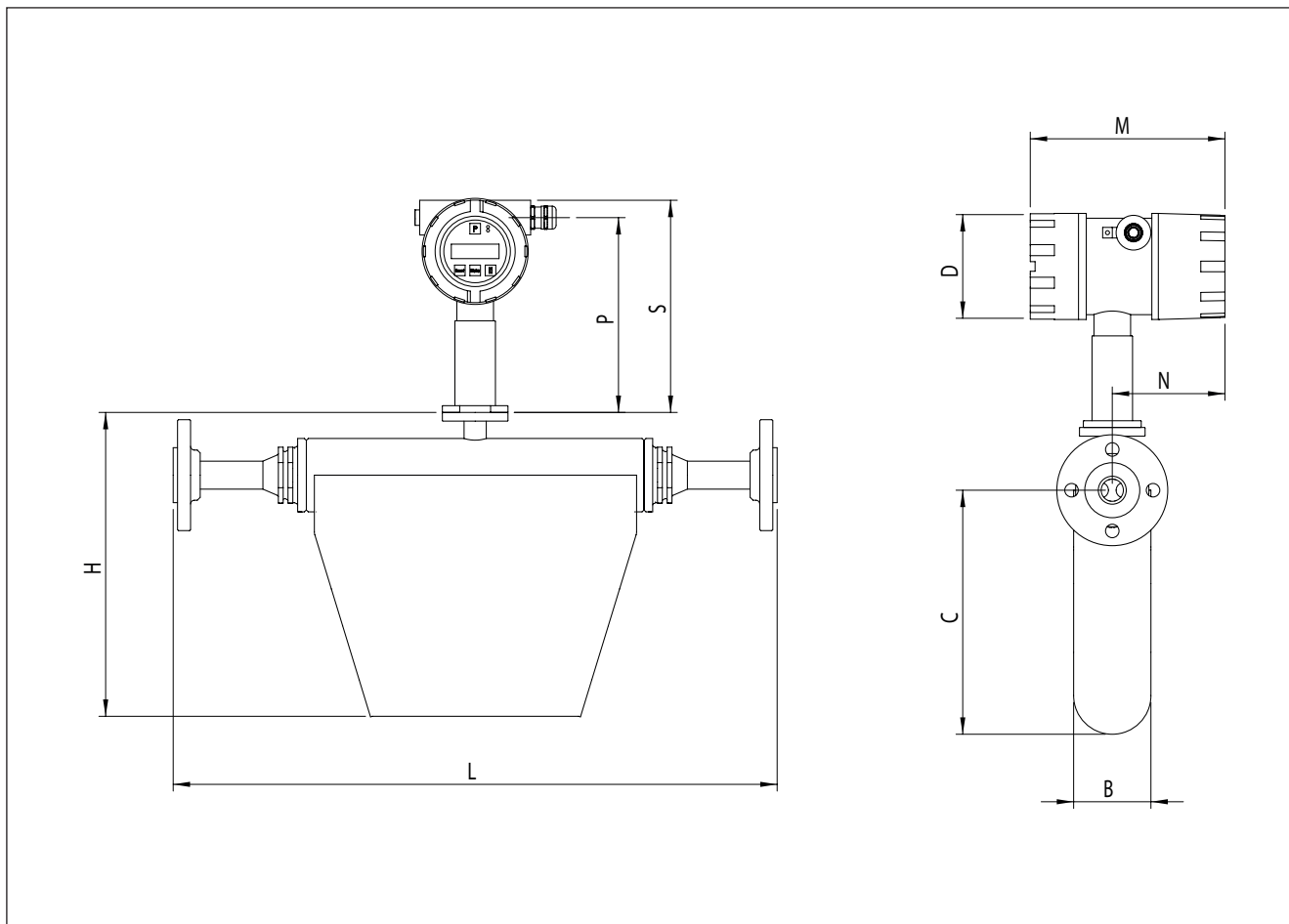
Чертеж (мм) TCM 28k до TCM 65k
