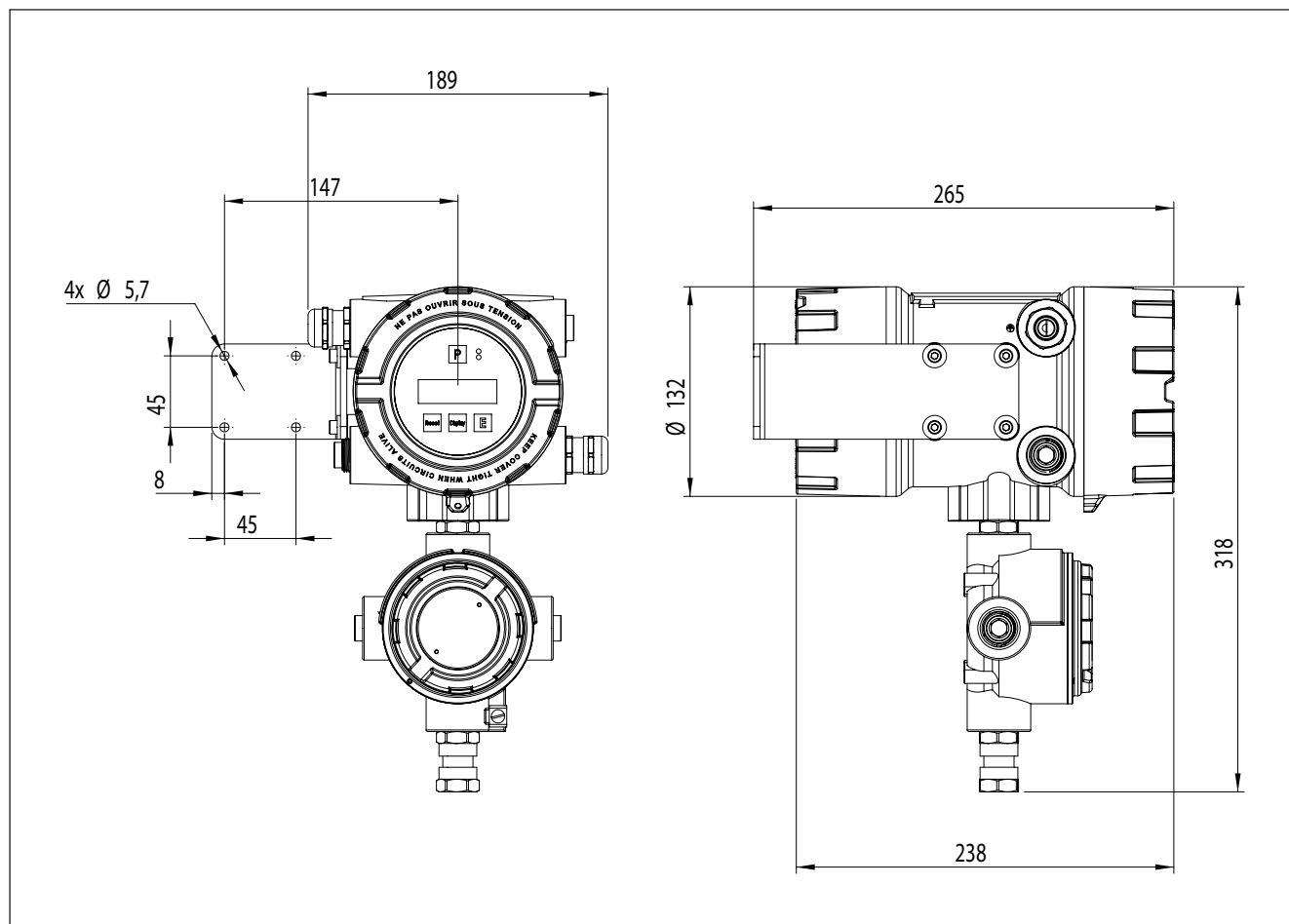
Чертеж (мм) TCE 80xx - E с клеммной коробкой
